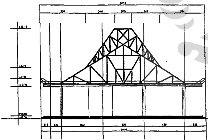
TAMPAK MUKA MUSHOLA
