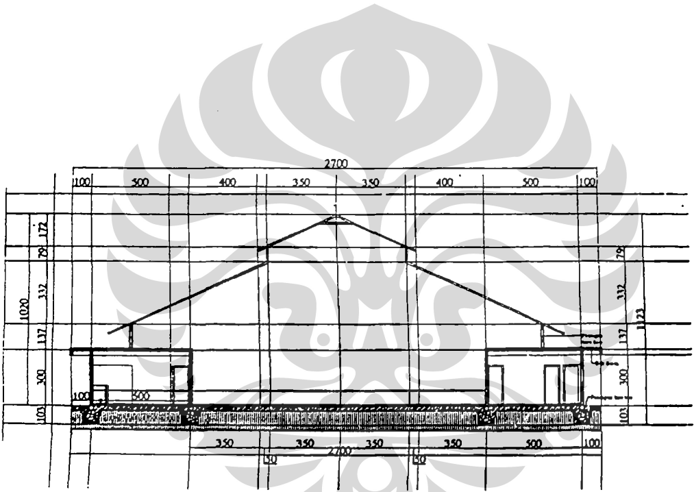
POTONGAN A-A
