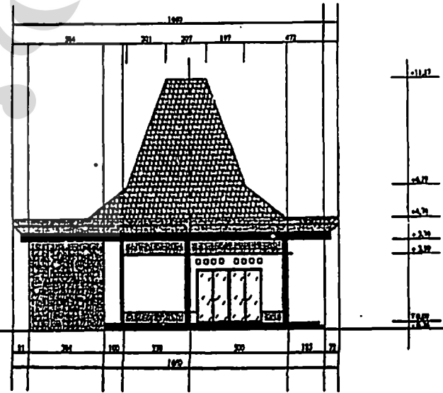
TAMPAK DARI SELATAN MUSHOLA
