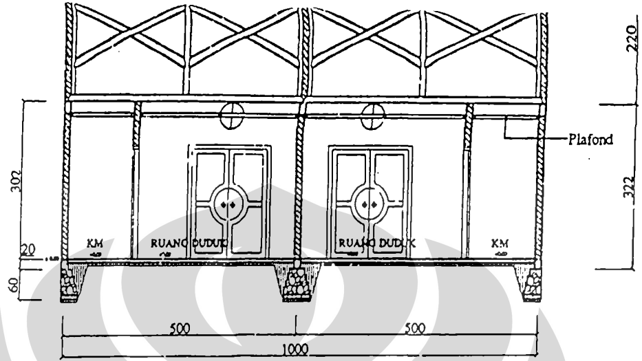
POTONGAN A - A SKALA 1:100
