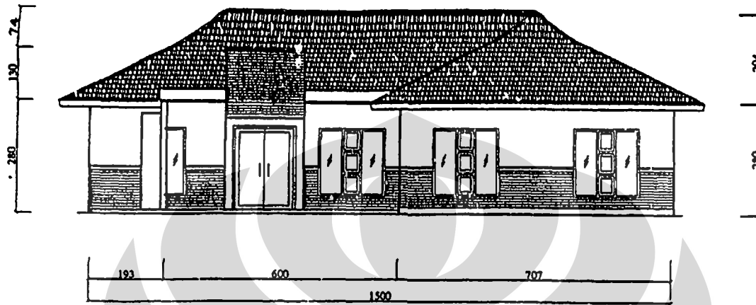
TAMPAK DEPAN SKALA 1:100
