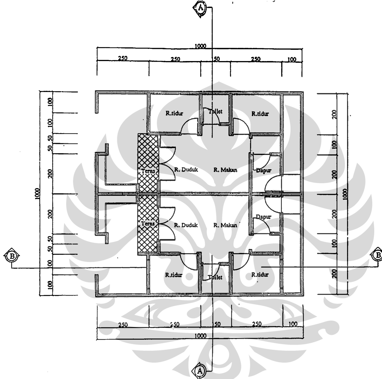
DENAH RUMAH JAGA SKALA 1 : 100
