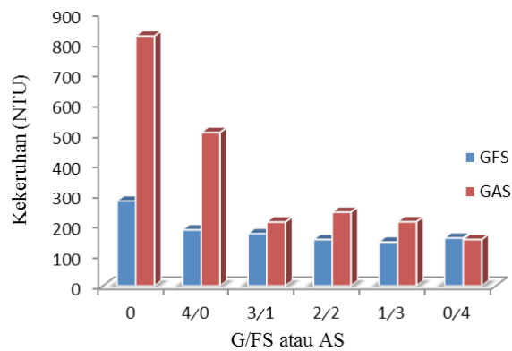
Gambar 3. Kekерuhan limbah cair pasca pengolahan
