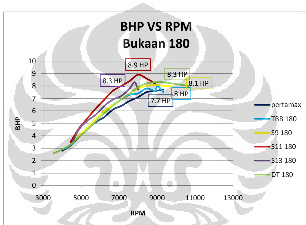
Grafik 5.1 Grafik perbandingan daya mesin pada bukaan katup 180^{\circ}
