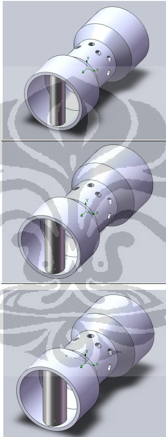
Gambar 2.17. Venturi Mixer 12 Lubang Menyilang Dengan Bluff Body Silinder Diameter 9mm (atas), 11mm (tengah), dan 13mm (bawah)
