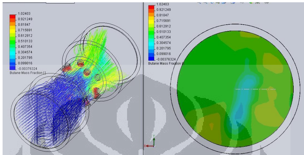
Gambar 2.5. Penyebaran Spesies Bluff Body Silinder Diameter 9 mm Pada Simulasi Cosmos Flow
