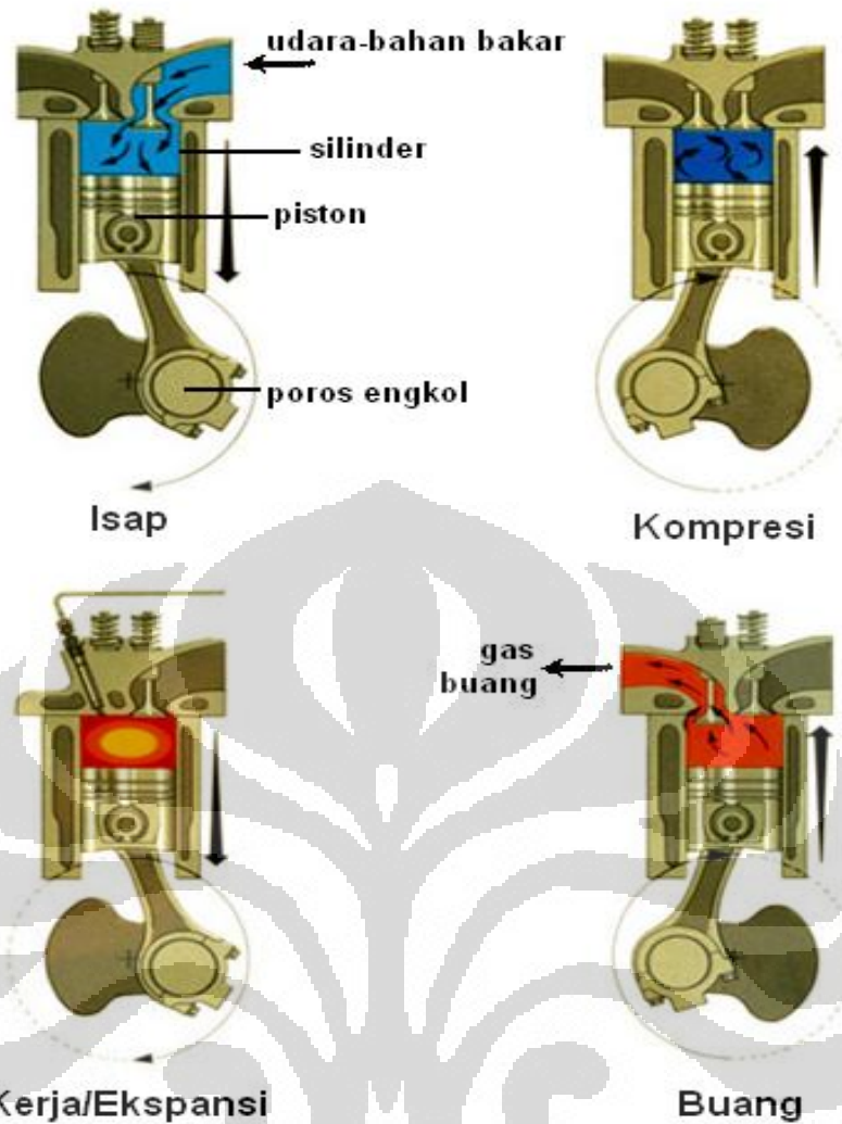
Gambar 2.1. Proses Kerja Motor Otto Empat Langkah
