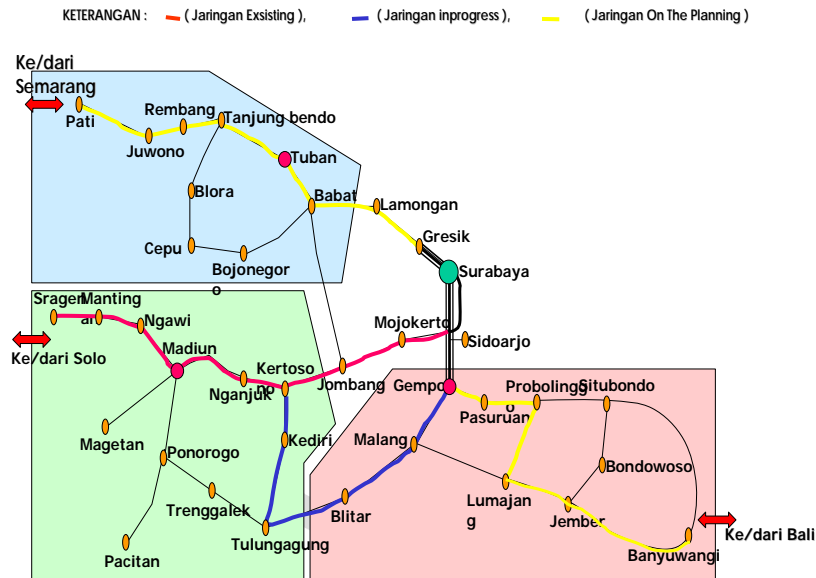
Gambar L- 28 Pengembangan Jaringan FO Indosat tahun 2008
