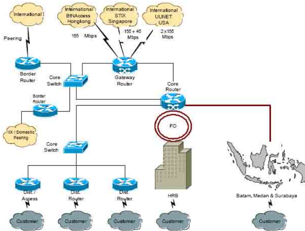
Gambar L- 37 Jaringan Global IM2
