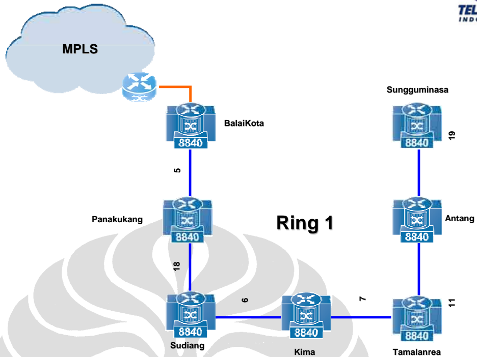
Gambar L- 17 Jaringan MEN TELKOM-STO Makassar
