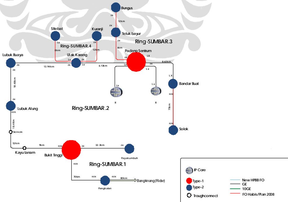
Gambar L- 4 Jaringan MEN TELKOM-STO Sumatera Barat
