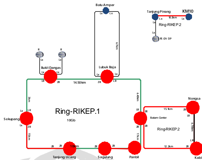
Gambar L- 5 Jaringan MEN TELKOM-STO Riau Daratan & Rikep
