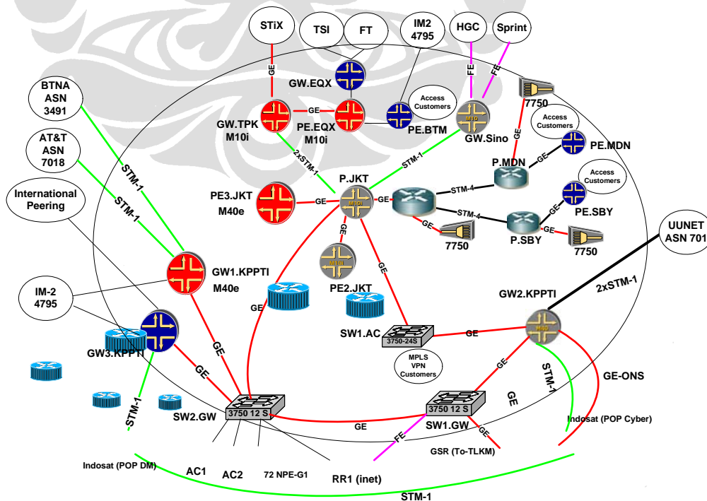
Gambar L- 29 Jaringan Global Indosat
