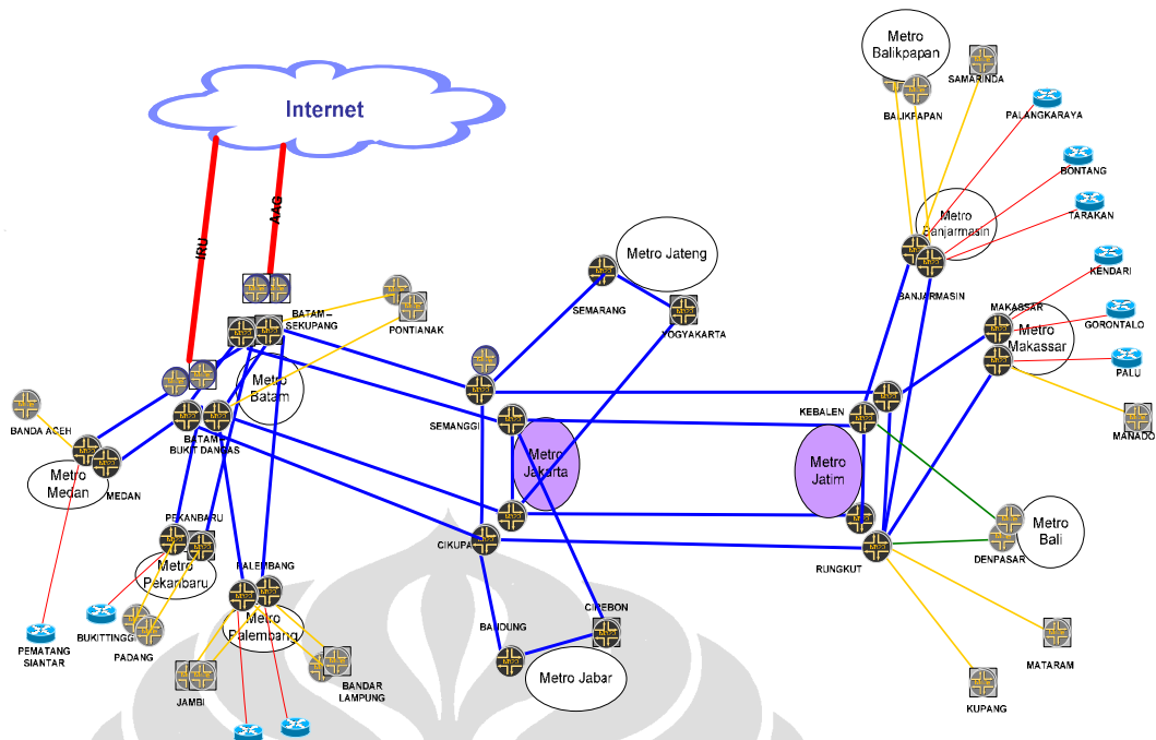
Gambar L- 19 Jaringan IP Core TELKOM
