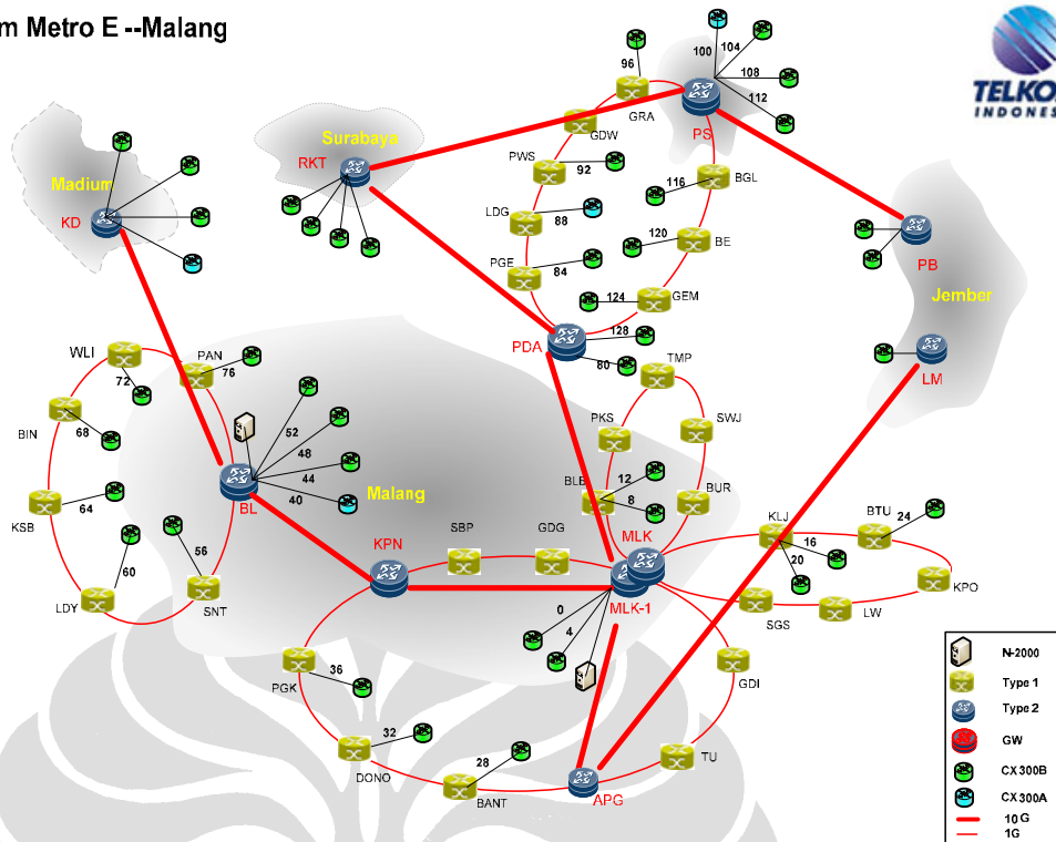
Gambar L- 13 Jaringan MEN TELKOM-STO Malang
