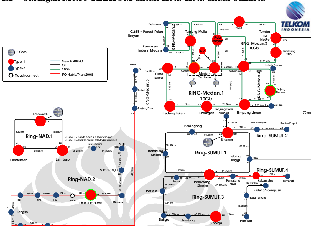
Gambar L- 3 Jaringan MEN TELKOM-STO Sumatera Bagian Utara
