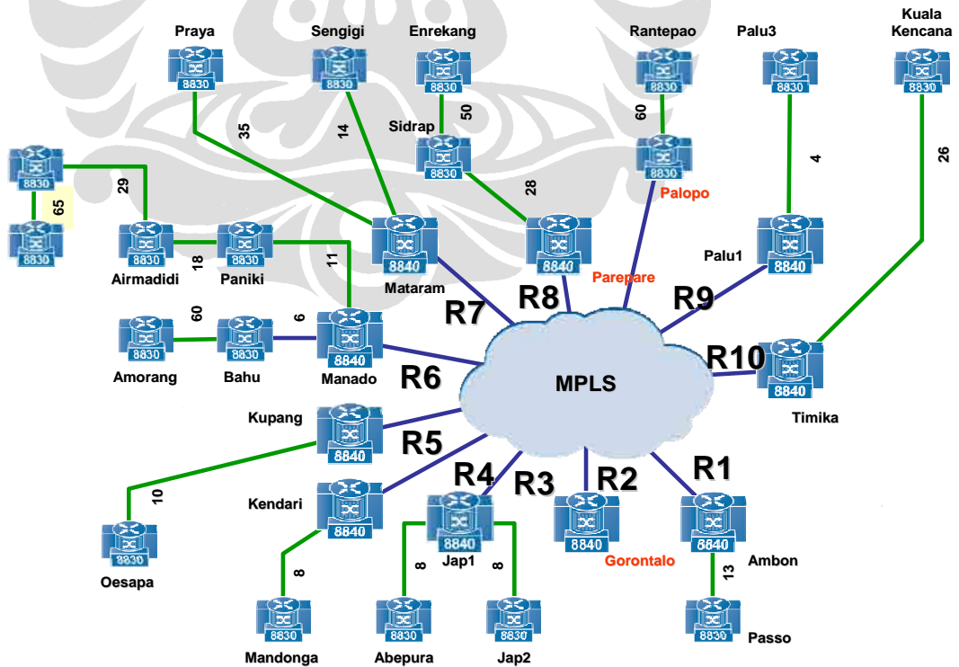
Gambar L- 18 Jaringan MEN TELKOM-STO KTI
