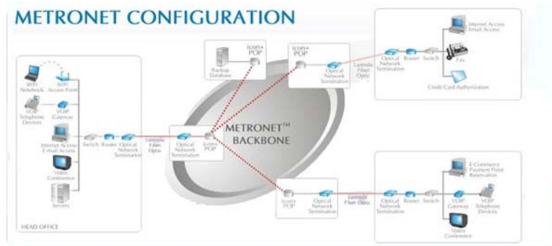
Gambar L- 60 Konfigurasi MetroNet
