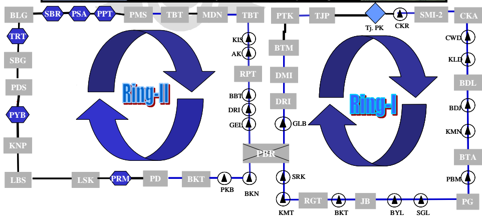
Gambar L- 23 Rencana Pengembangan Jasuka TELKOM 2008
