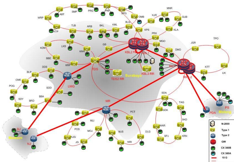
Gambar L- 12 Jaringan MEN TELKOM-STO Surabaya
