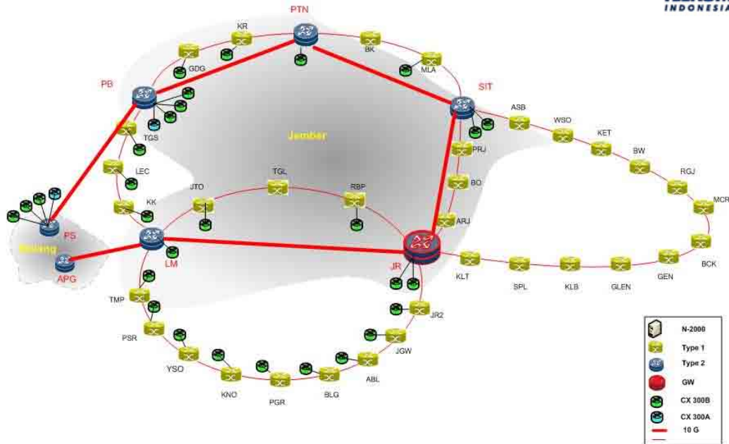
Gambar L- 15 Jaringan MEN TELKOM-STO Jember
