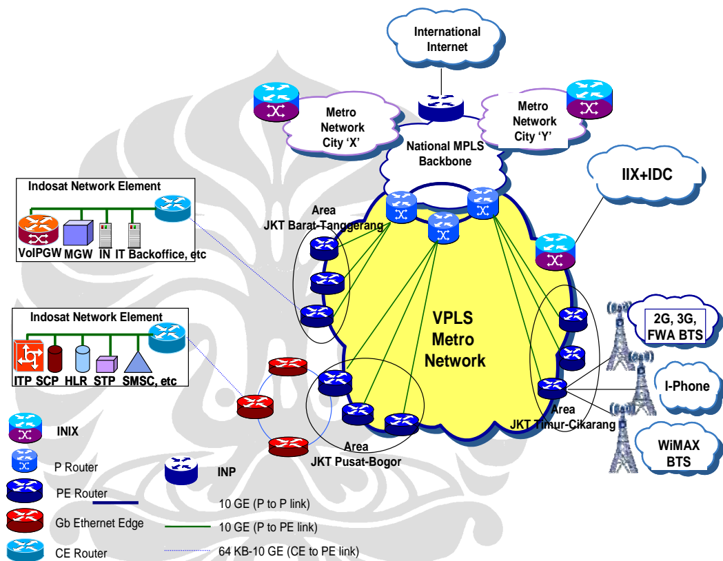
Gambar L- 25 Jaringan Metro Ethernet Indosat Area Jakarta
