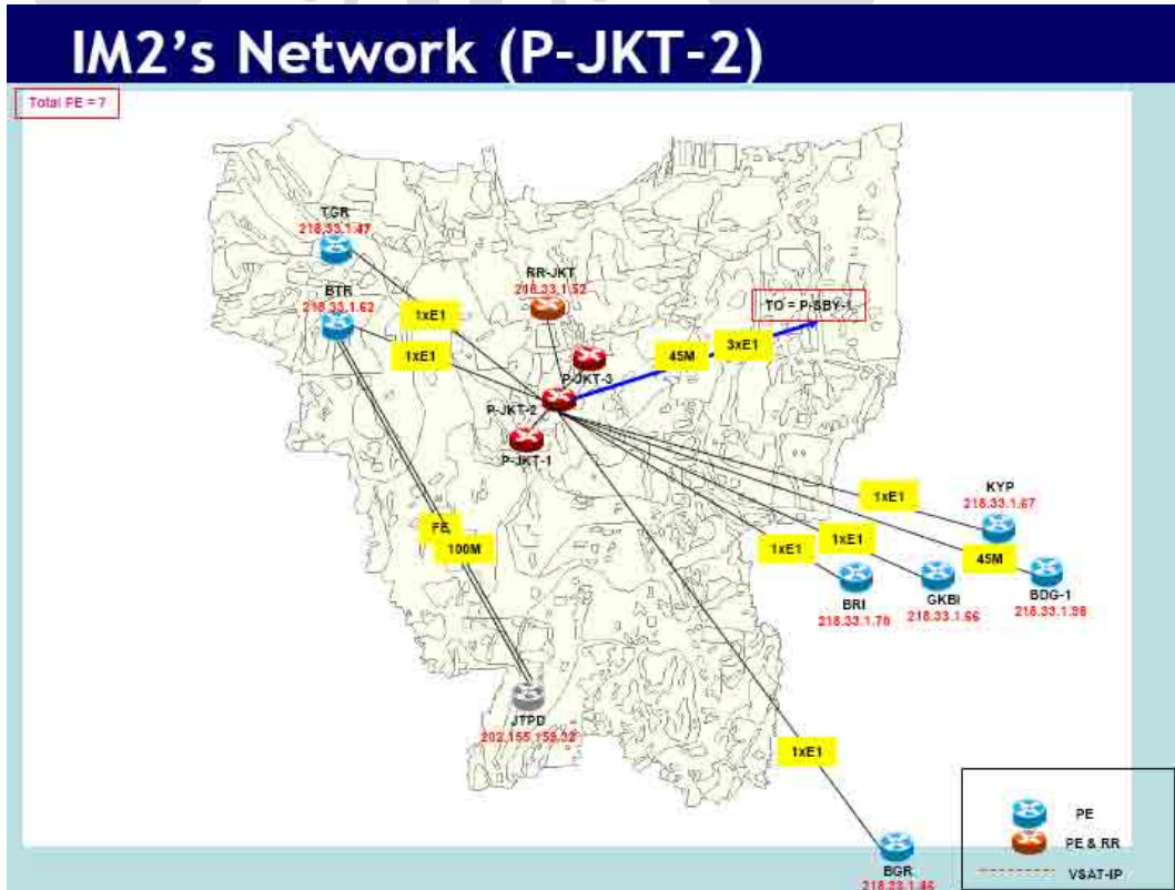
Gambar L- 33 Jaringan Metro IM2 P-JKT-2
