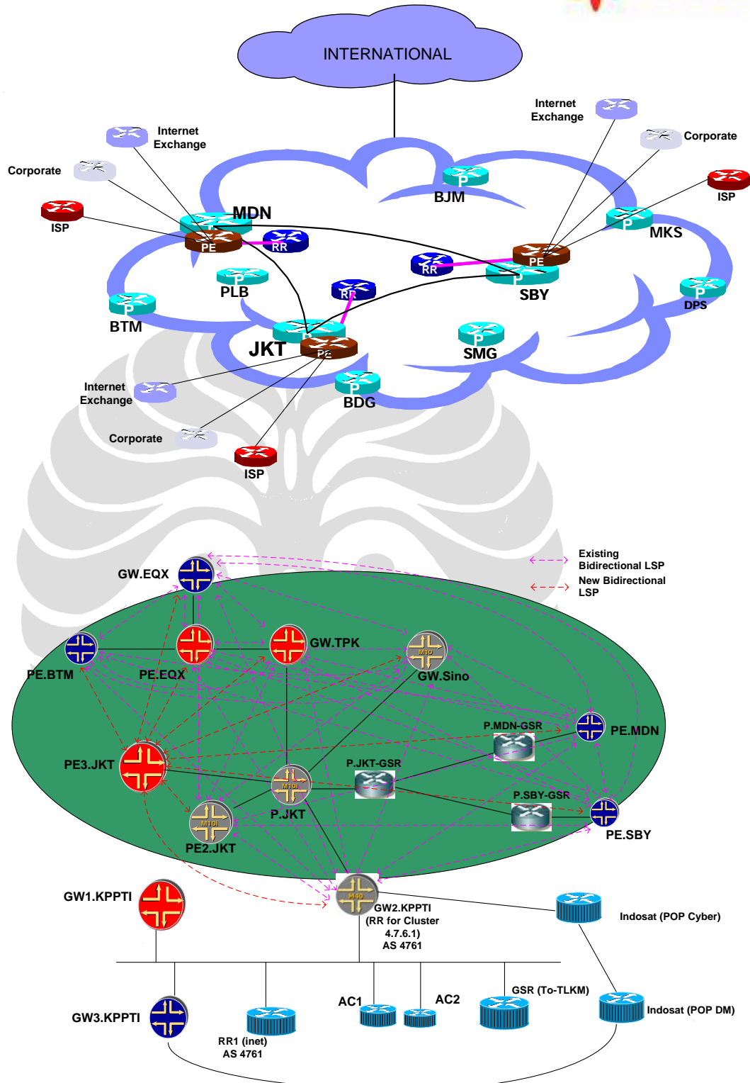
Gambar L- 26 Jaringan IP-Core Nasional Indosat
