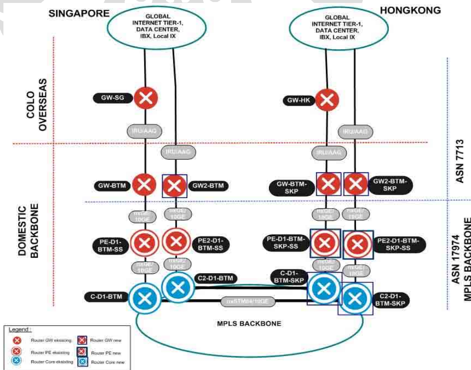
Gambar L- 20 Jaringan IP Core Global TELKOM
