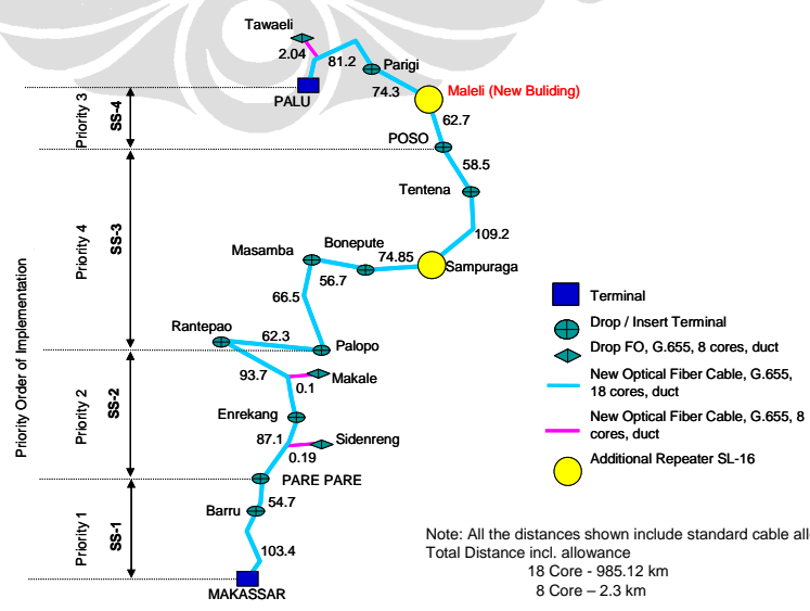
Gambar L- 24 Rencana pengembangan FO TELKOM wilayah Kalimantan & Sulawesi 2008
