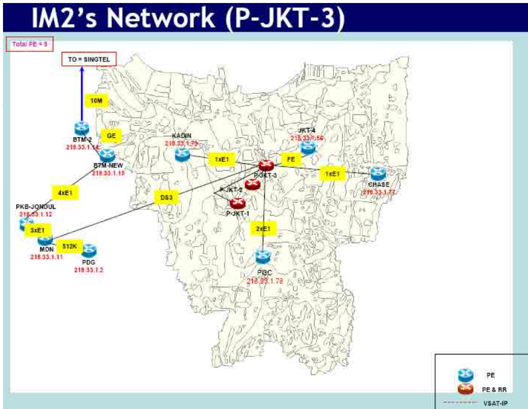
Gambar L- 34 Jaringan Metro IM2 P-JKT-3
