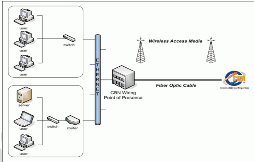
Gambar L- 64 Tipikal jaringan metro CBN
