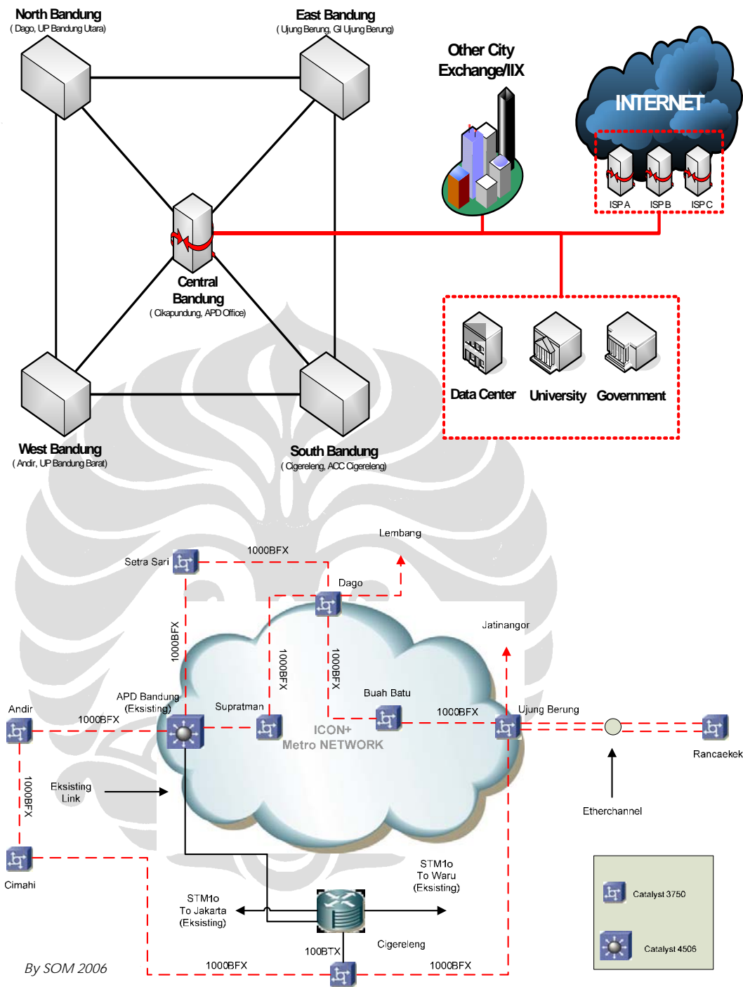
Gambar L- 59 Tipikal jaringan Metro ICON+ Area Bandung
