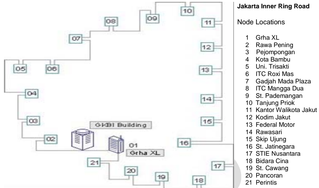
Gambar L- 42 Konfigurasi dan lokasi XL-HRB Metro Area Jakarta
