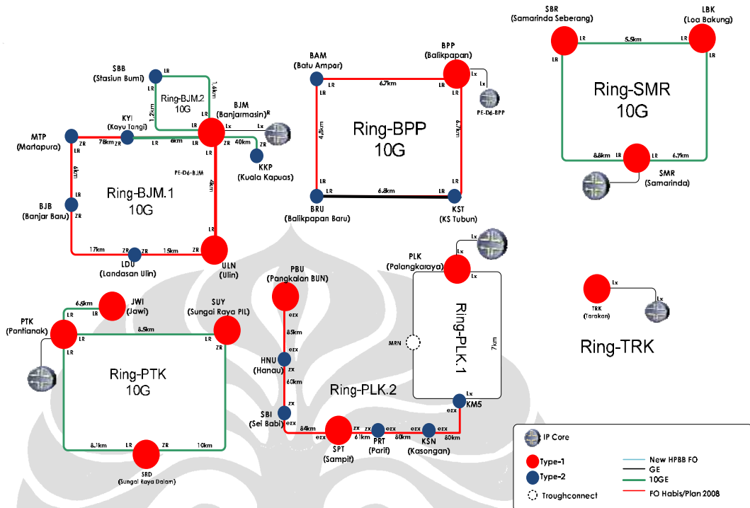
Gambar L- 8 Jaringan MEN TELKOM-STO Kalimantan
