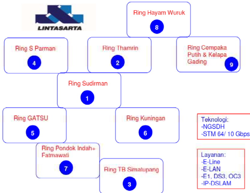
Gambar L- 39 Konfigurasi Ring Metro Lintasarta
