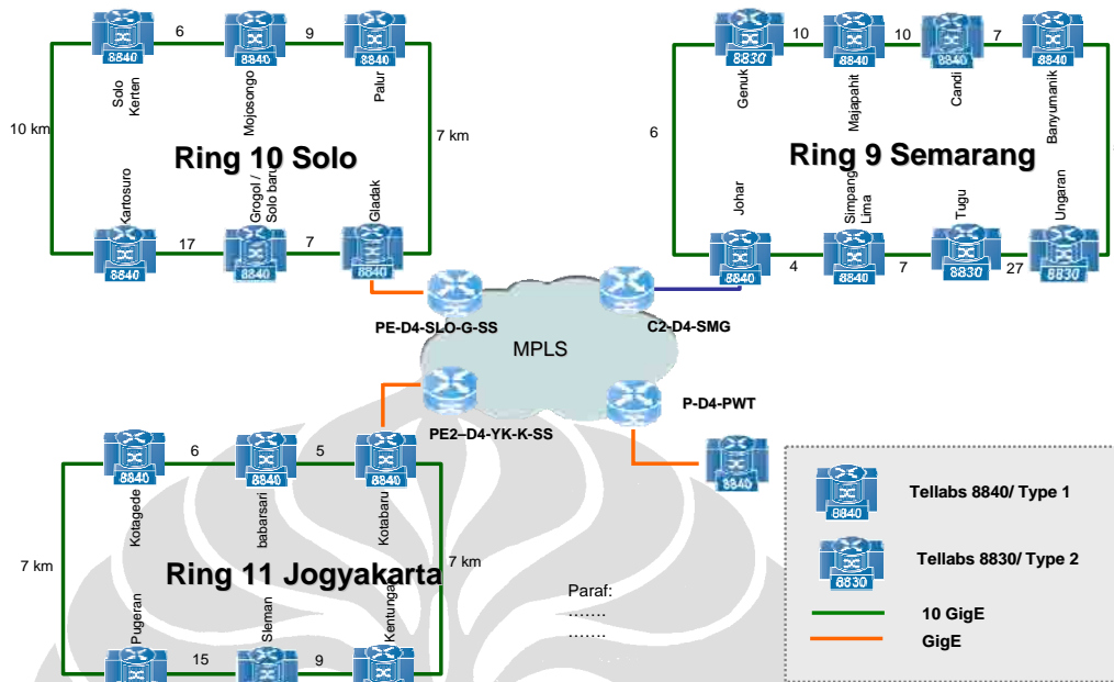
Gambar L- 10 Jaringan MEN Jawa Tengah
