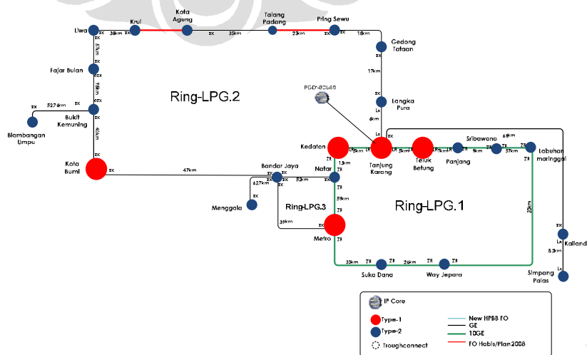
Gambar L- 7 Jaringan MEN Lampung
