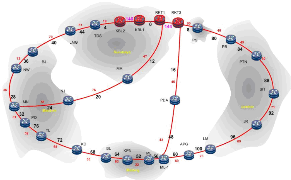
Gambar L- 11 Jaringan MEN Regional TELKOM-STO DIVRE 5 Jawa Timur
