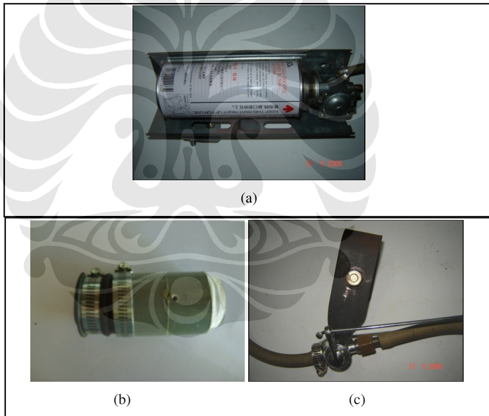
Gambar 3.2. (a) Kompor gas portabel, (b) Venturi mixer dan (c) Katup penghubung
