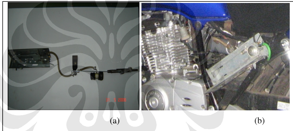
Gambar 3.1. (a) Sistem penyaluran gas LPG model lama (b) Penempatan sistem penyaluran gas LPG pada sepeda motor model baru ( venturi mixer)
