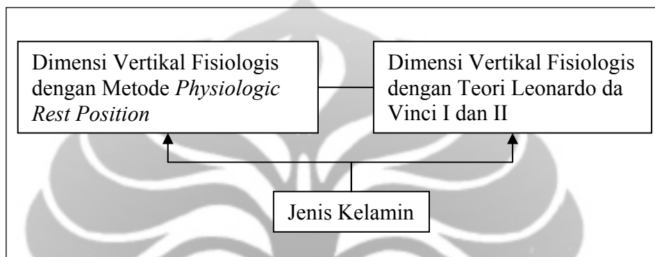
Diagram 3.1 Kerangka Konsep
