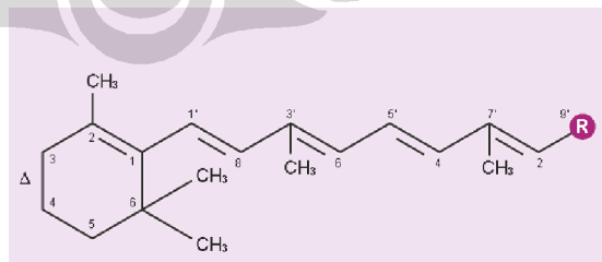
Gambar 2. Rumus Struktur Vitamin A
