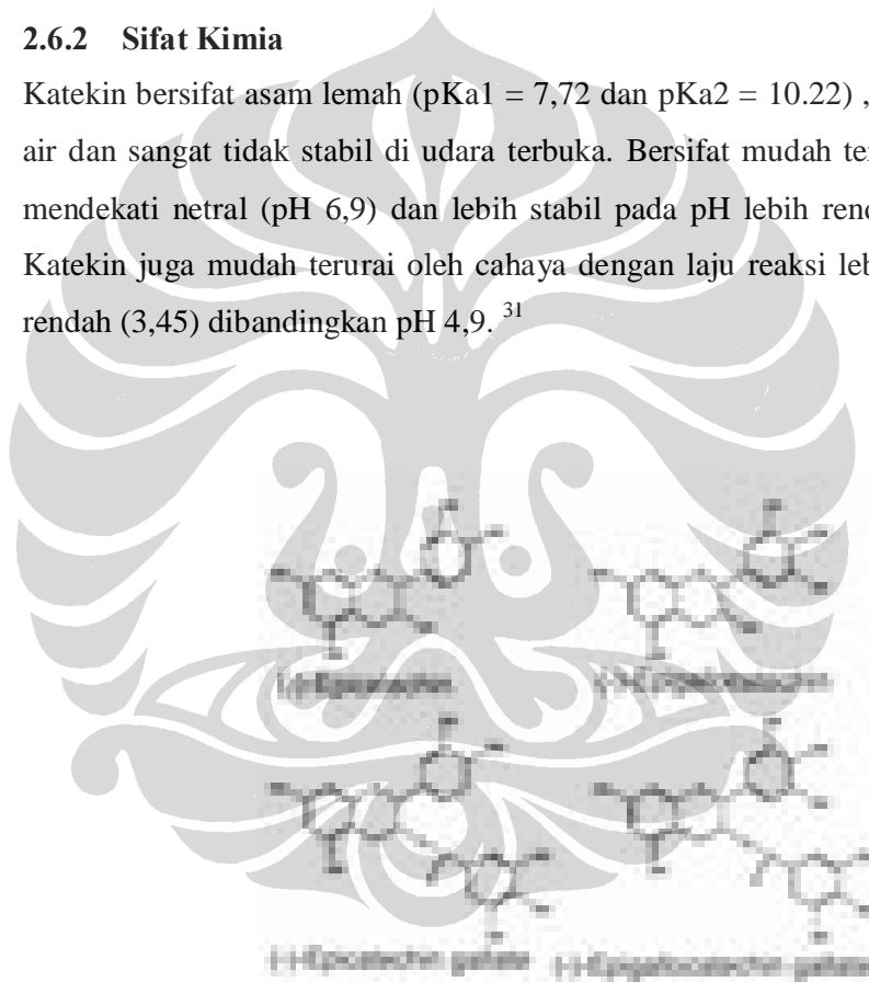
Gambar 4. Rumus Struktur Katekin 32
