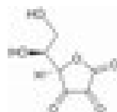
Asam L-dehidro askorbat (bentuk teroksidasi).
