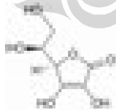
Asam L-Askorbat (Bentuk tereduksi)
