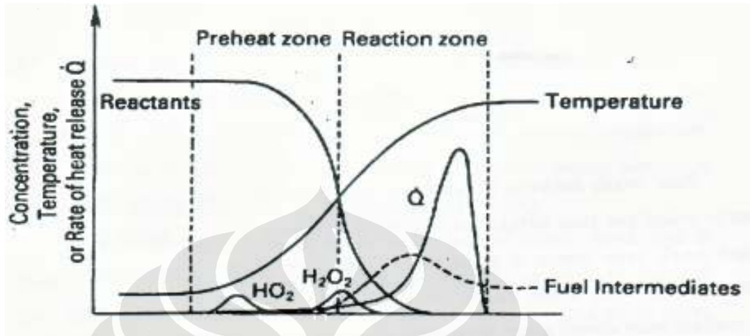
1Gambar 2.2 Profil Nyala Api
