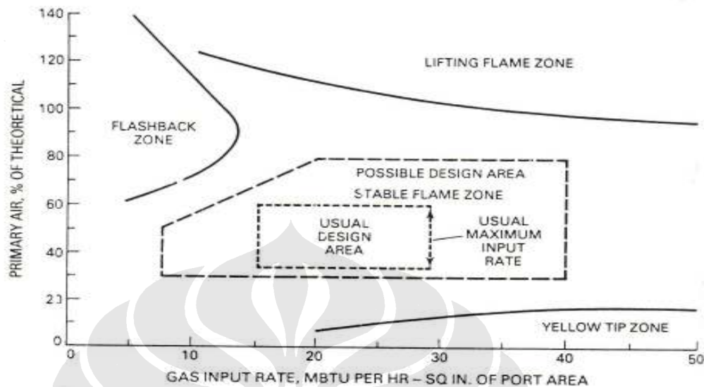
Gambar 2.5 Diagram stabilitas flashback , lift-off , dan yellow tipping untuk bahan bakar gas industri
