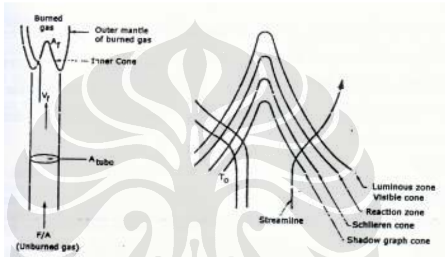
2Gambar 2.3 Struktur Nyala Api Premix [15]
