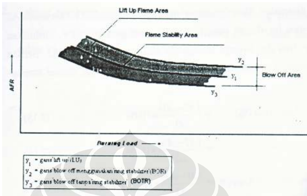
4Gambar 2.6 Grafik Perbandingan AFR dan BL
