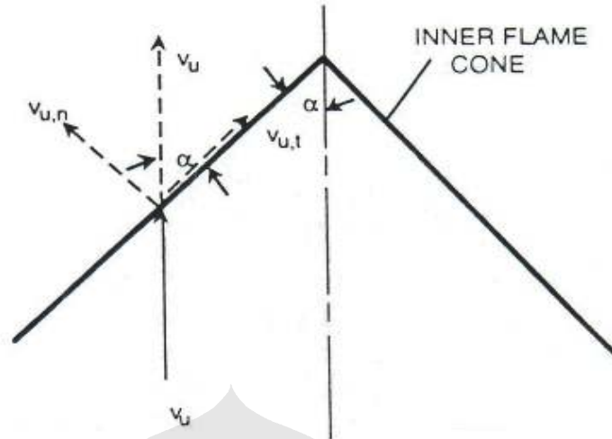
3Gambar 2.4 Vektor Diagram Kecepatan Nyala Laminar [18]
