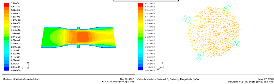
Venturi mixer 4
