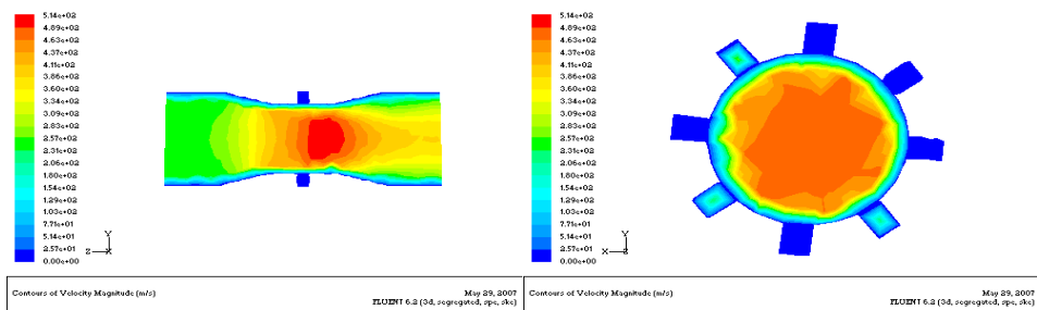
Venturi mixer 12
