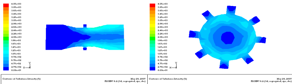
Venturi mixer 12
