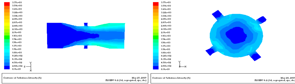
Venturi mixer 8
