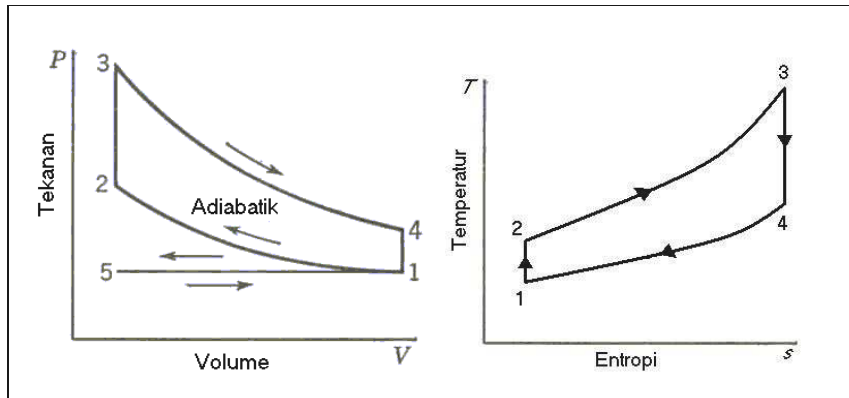
Gambar 2.2. Diagram P-V Dan T-S Ideal Motor Otto 4 Langkah
