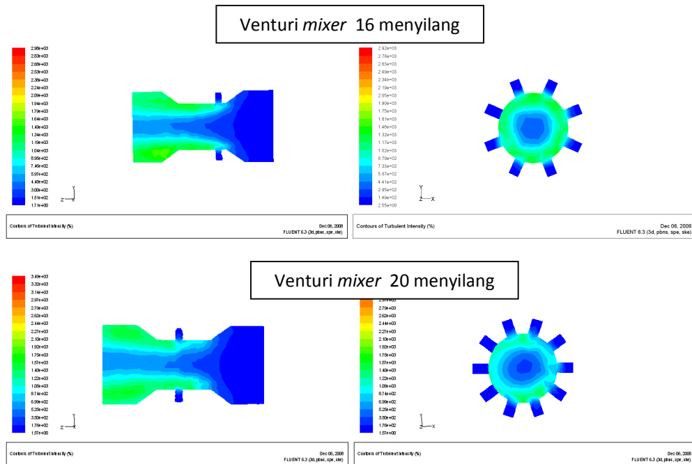
Gambar 2.7 Kontur Turbulensi Pada Simulasi CFD
