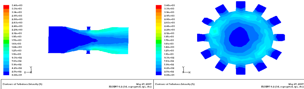
Venturi mixer 12
