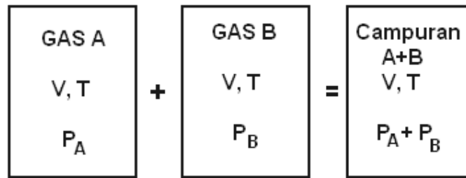
Gambar 2.4. Hukum Dalton
