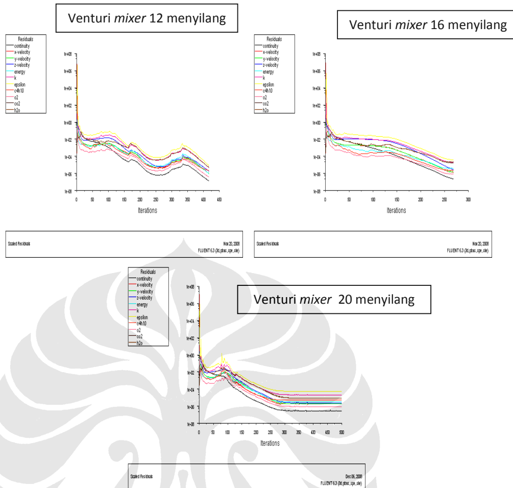
Gambar 2.5. Grafik iterasi
