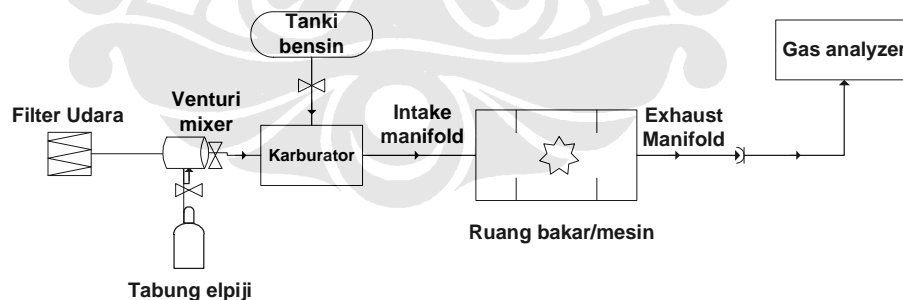
Gambar 3.4 Skema Pencampuran Bahan Bakar
