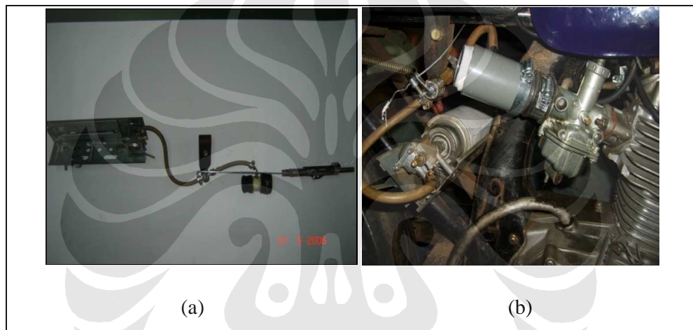
Gambar 3.1. (a) Sistem Penyaluran Gas LPG Model Lama, (b) Penempatan Sistem Penyaluran Gas LPG Pada Sepeda Motor Model Baru ( Venturi Mixer)
