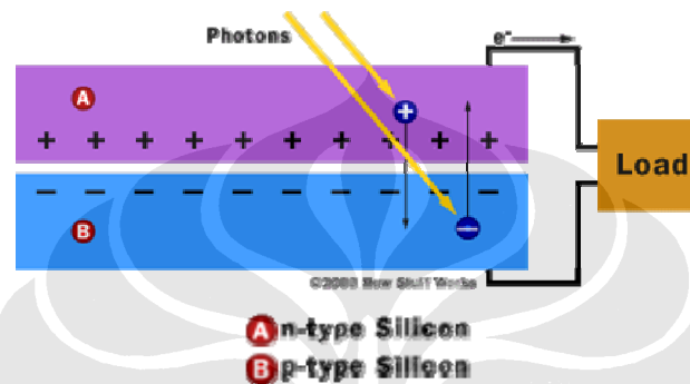
Gambar 2.6 Aliran Elektron Pada Sel Surya [3]
