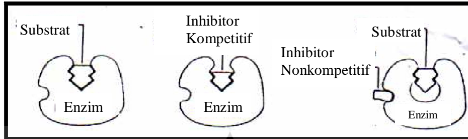
Gambar 2.2 Perbedaan struktur penghambatan kompetitif dan nonkompetitif
