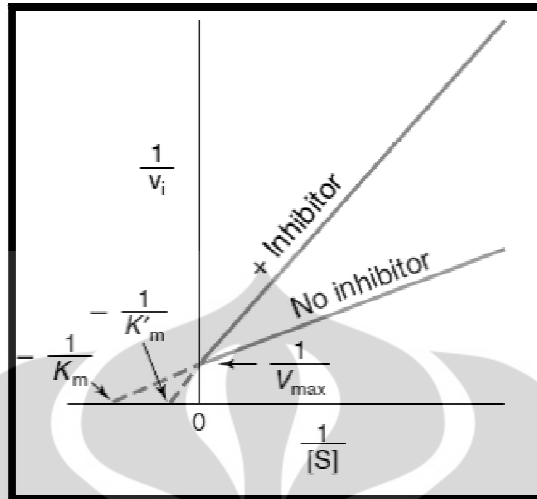
Gambar 2.5 Plot Lineweaver-Burk untuk inhibisi kompetitif
