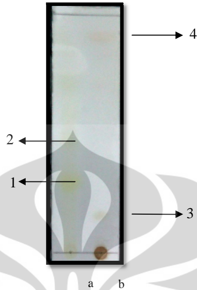
Gambar 4.10 Kromatogram antrakuinon (a) fraksi G (b) standar (Rhei Radix) secara visual setelah disemprot larutan KOH 8% dengan eluen n-heksana : etil asetat (7 : 3)
