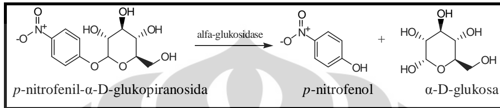
Gambar 2.8 Persamaan reaksi enzimatik \alpha -glukosidase dan p -nitrofenil- \alpha -D-glukopiranosida
