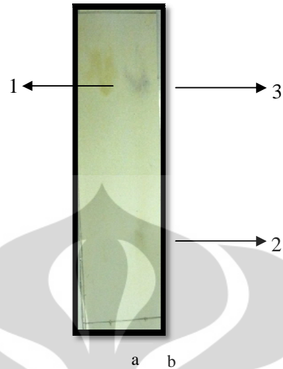
Gambar 4.8 Kromatogram tanin (a) fraksi G (b) standar ( Theae Folium ) secara visual setelah disemprot larutan \text{FeCl}_3 dengan eluen butanol : asam asetat glasial : akuades (4:1:5)
