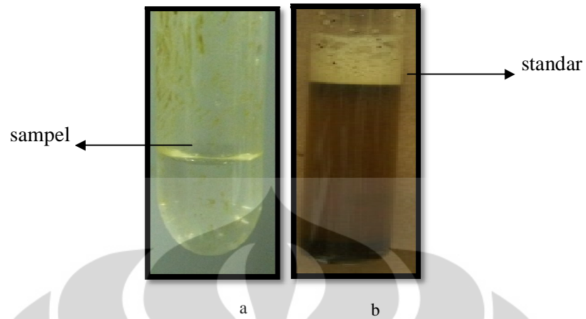
Gambar 4.14 Identifikasi saponin (a) fraksi G (b) standar ( Ortosiphon Folium ) dengan pengocokan dan penambahan asam klorida
