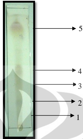
Gambar 4.4 Pola kromatogram fraksi G secara visual setelah disemprot larutan asam sulfat 10% dan dipanaskan dengan eluen n-heksana : etil asetat (7:3)
