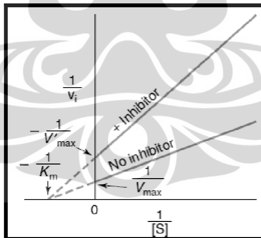
Gambar 2.6 Plot Lineweaver-Burk untuk inhibisi nonkompetitif
