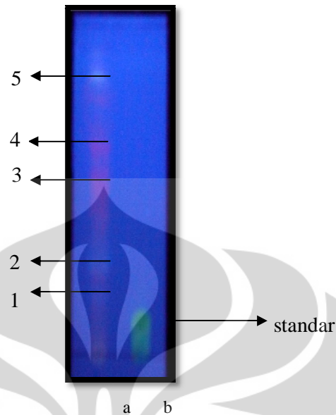
Gambar 4.6 Kromatogram flavonoid (a) fraksi G (b) standar (kuersetin) [di bawah UV 366 nm] setelah disemprot larutan \text{AlCl}_3 dengan eluen n-heksana : etil asetat (7 : 3)
