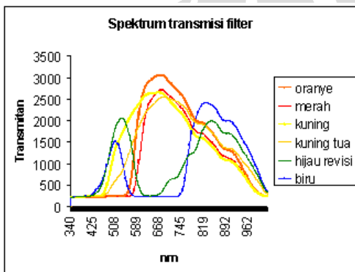
Gambar 4. Spektrum transmisi dari beberapa filter
