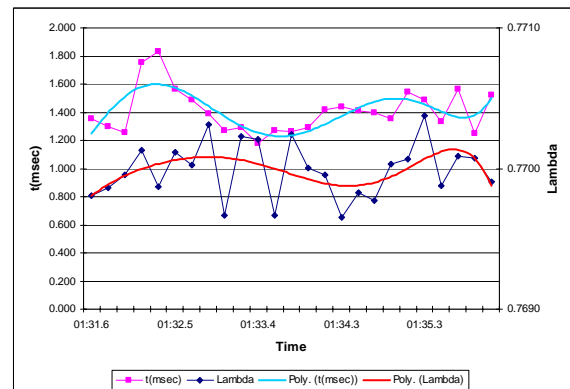
Gambar 9. Grafik durasi injektor dan lambda saat stasioner kecepatan rendah
