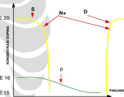
Gambar 2. Bentuk doping dari unilateral GCMOSFET
