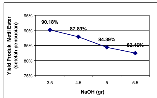
Gambar 3. Grafik Yield Produk Metil Ester (setelah pencucian) vs NaOH
