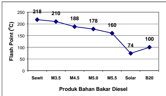
Gambar 7. Grafik Flash Ponit vs Produk bahan bakar diesel
