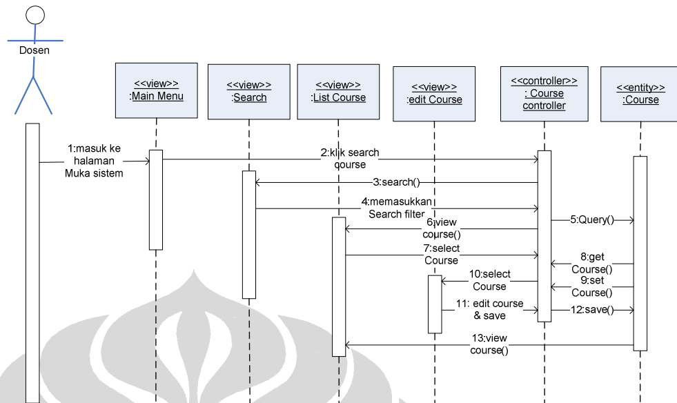
Gambar 56. Sequence diagram untuk use case Edit Course
