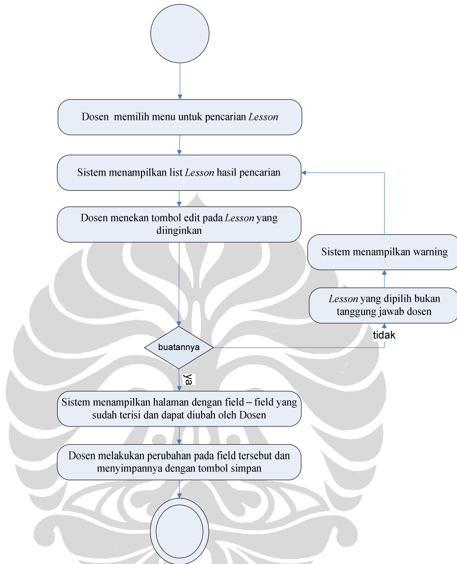
Gambar 35. Activity diagram untuk use case Edit Lesson
