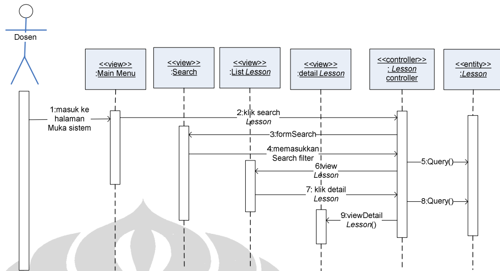
Gambar 54. Sequence diagram untuk use case View Detail Lesson
