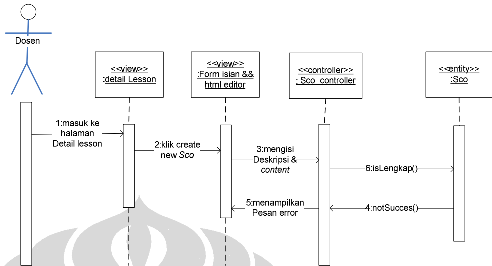
Gambar 46. Sequence diagram untuk use case New Sco
