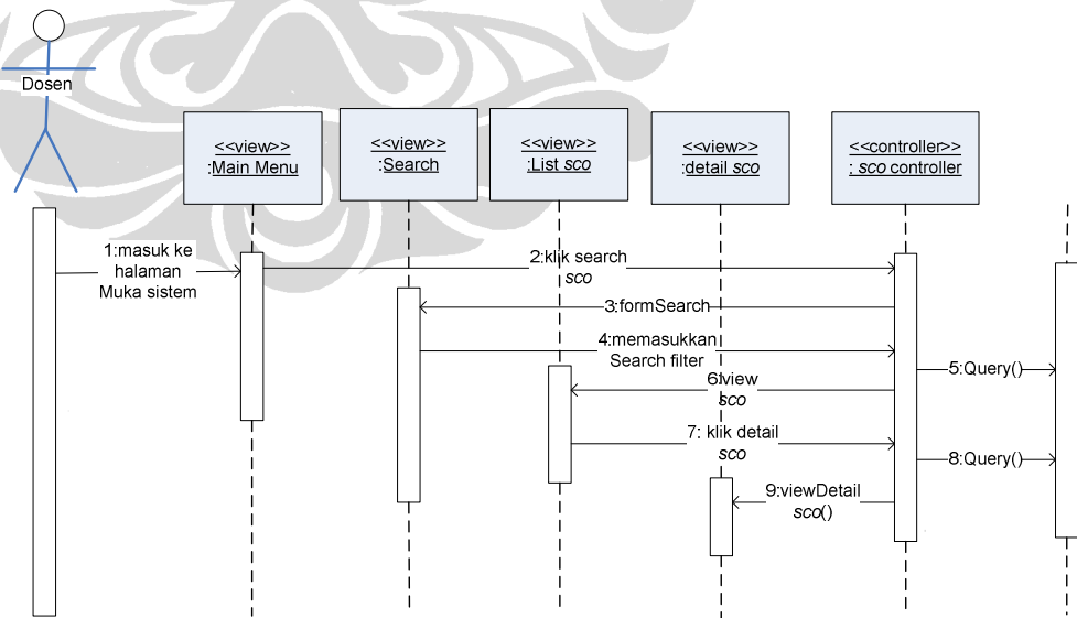
Gambar 53. Sequence diagram untuk use case View Detail Sco
