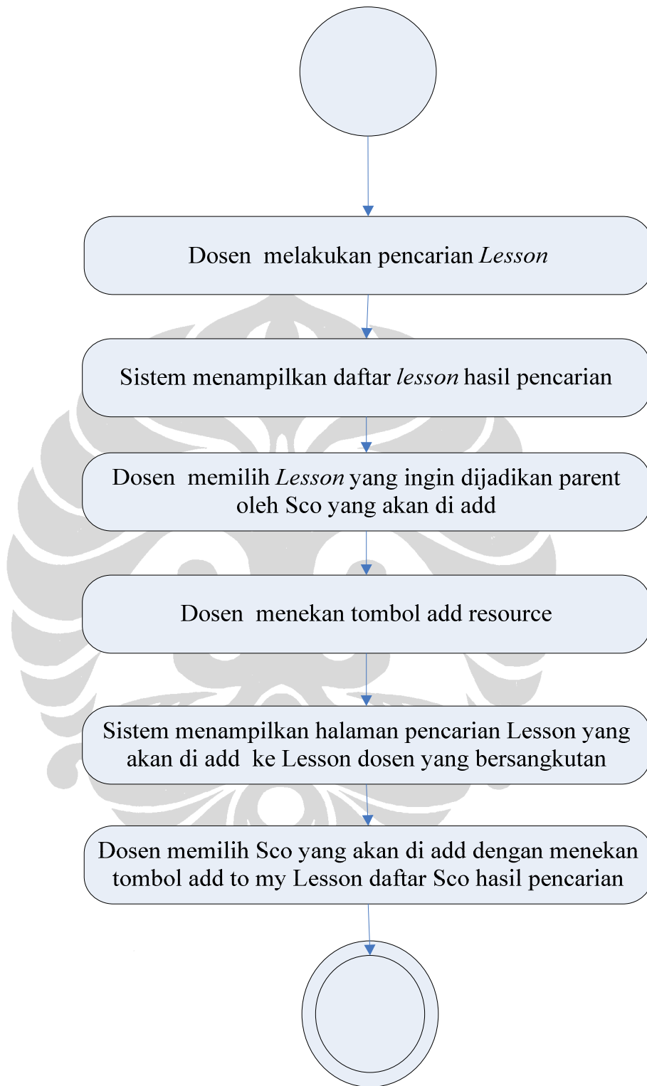
Gambar 25. Activity diagram untuk use case Add Sco From Other Course
