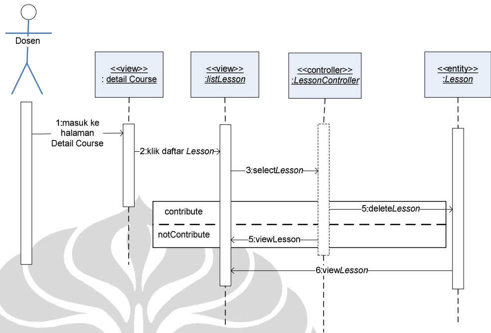
Gambar 62. Sequence diagram untuk use case delete Lesson
