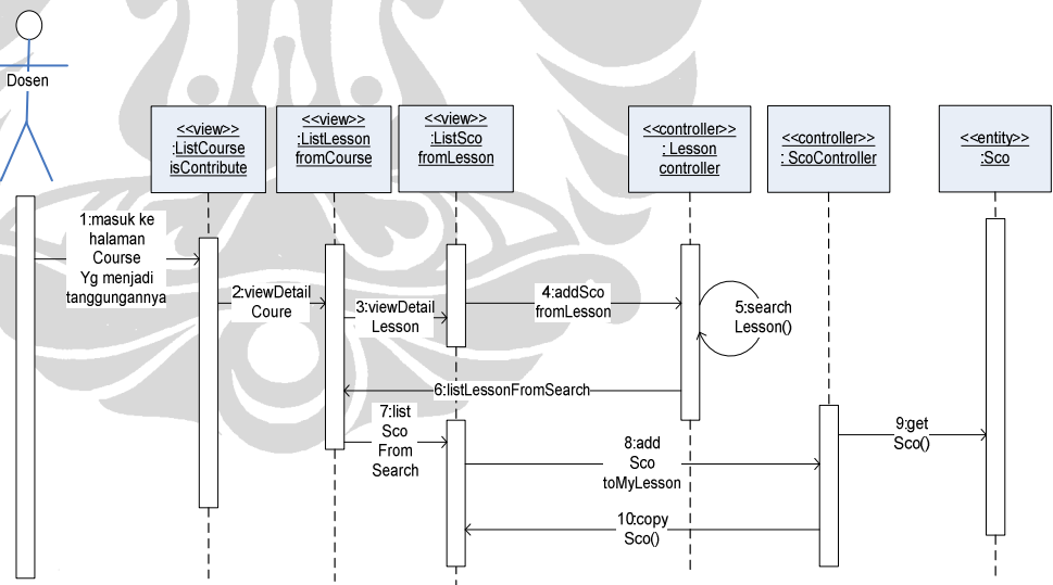
Gambar 47. Sequence diagram untuk use case Add Sco
