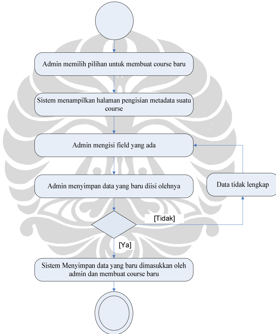
Gambar 22. Activity diagram untuk use case New Course
