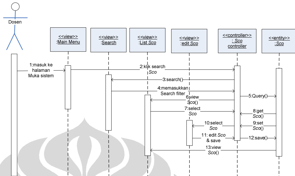
Gambar 58. Sequence diagram untuk use case Edit Sco
