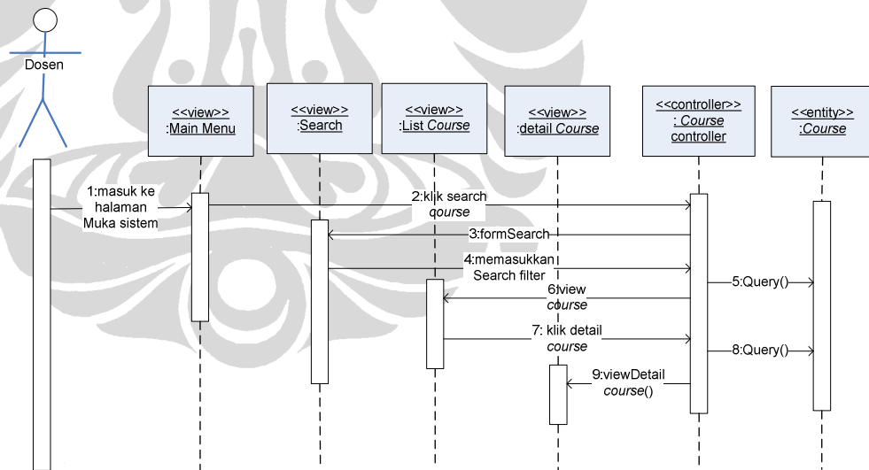
Gambar 55. Sequence diagram untuk use case View Detail Course
