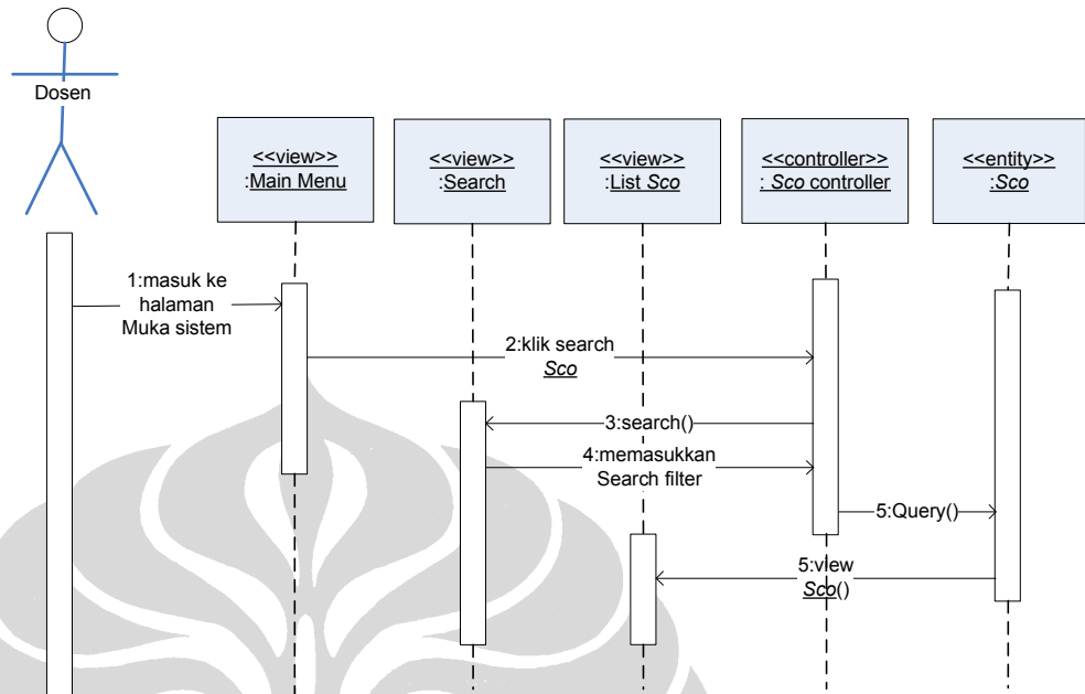
Gambar 50. Sequence diagram untuk use case Search Sco
