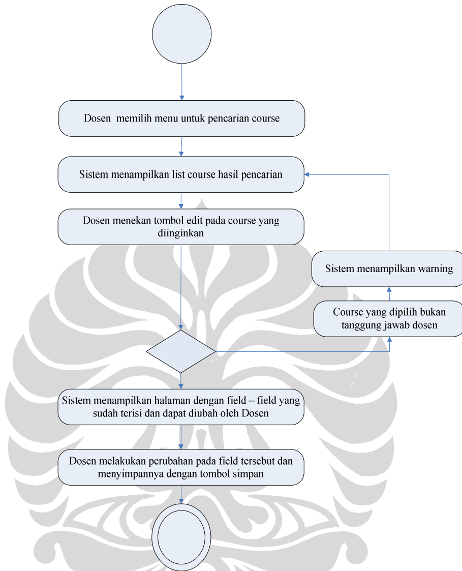
Gambar 36. Activity diagram untuk use case Edit Course
