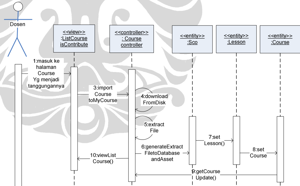
Gambar 65. Sequence diagram untuk use case Import Course
