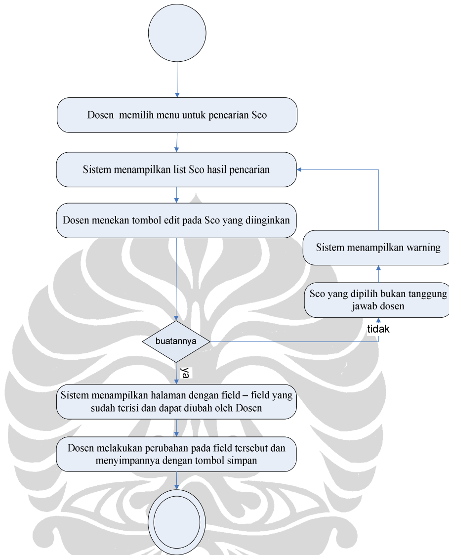
Gambar 34. Activity diagram untuk use case Edit Sco
