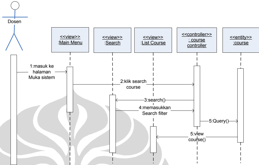
Gambar 52. Sequence diagram untuk use case Search Course
