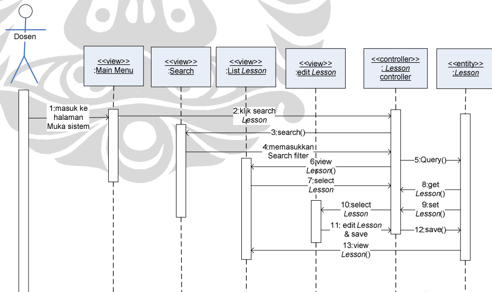
Gambar 57. Sequence diagram untuk use case Edit Lesson
