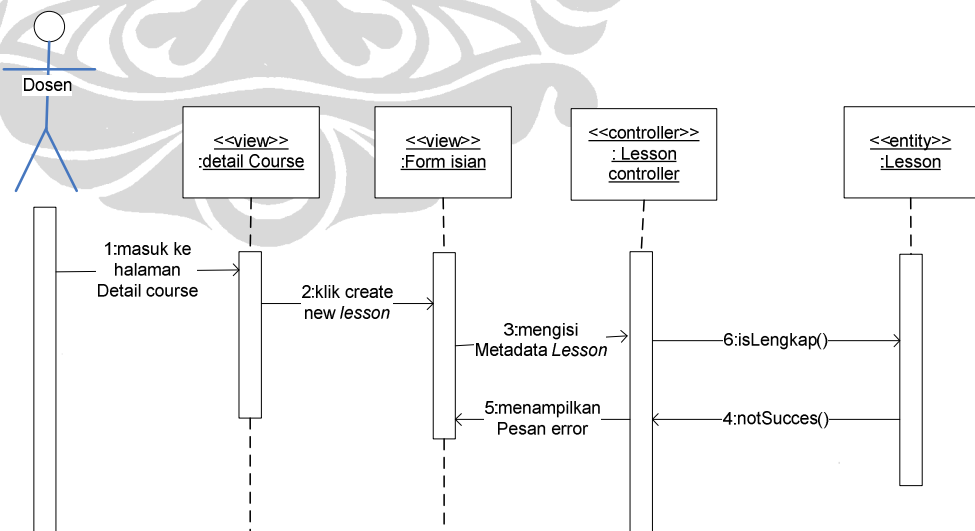
Gambar 45. Sequence diagram untuk use case New Lesson
