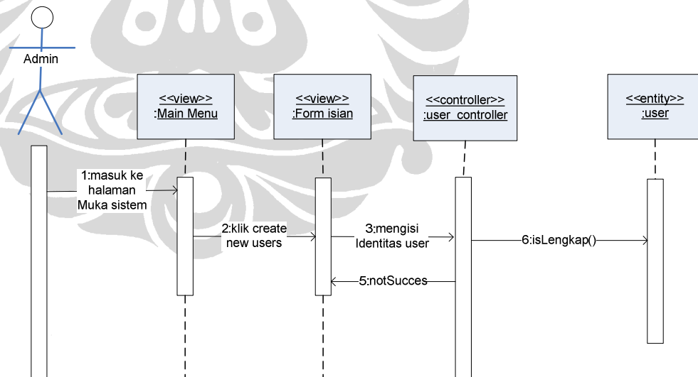
Gambar 59. Sequence diagram untuk use case Create New User
