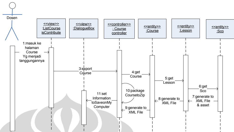
Gambar 64. Sequence diagram untuk use case Export course
