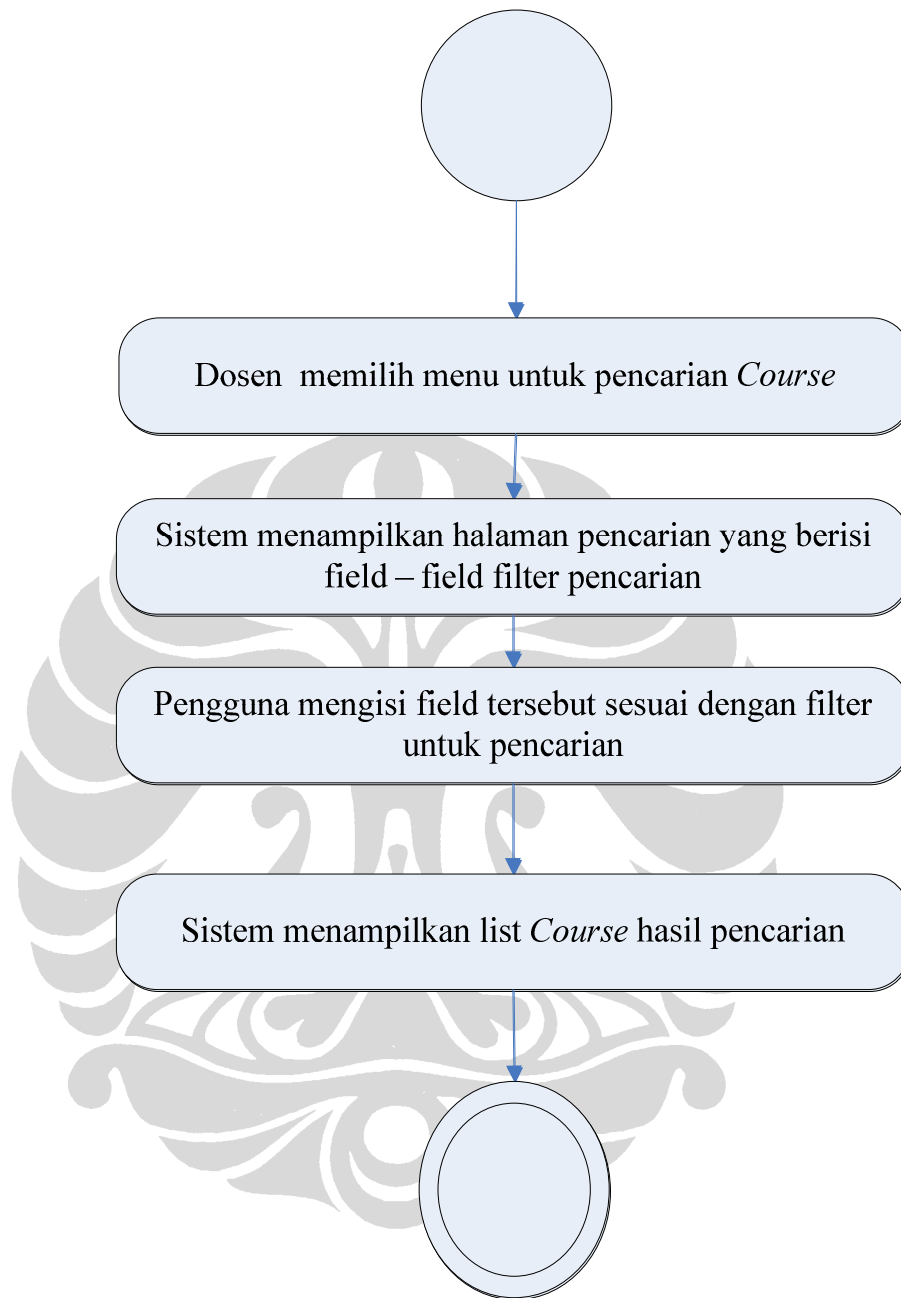
Gambar 28. Activity diagram untuk use case Search course
