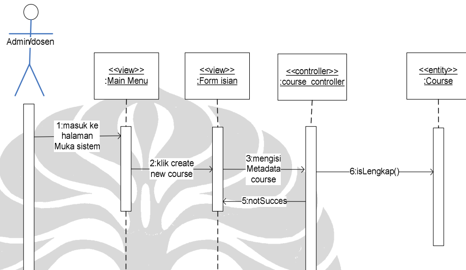
Gambar 44. Sequence diagram untuk use case New Course
