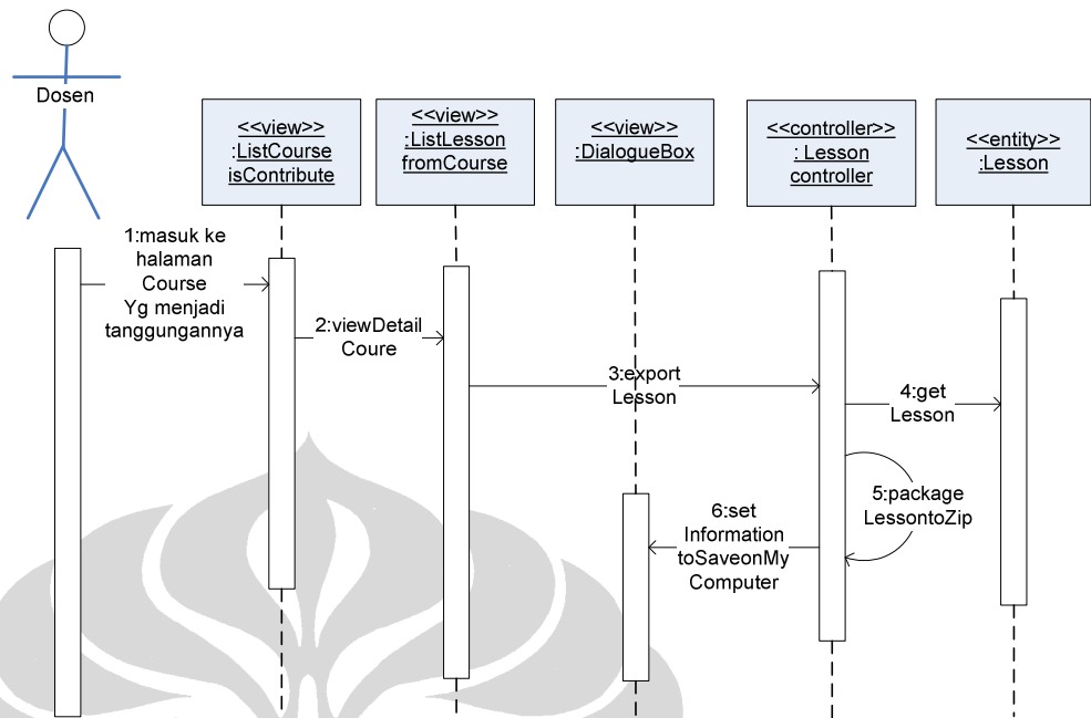
Gambar 48. Sequence diagram untuk use case Export Lesson
