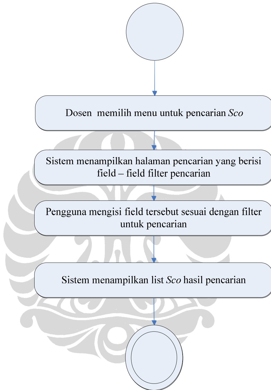
Gambar 30. Activity diagram untuk use case Search Sco
