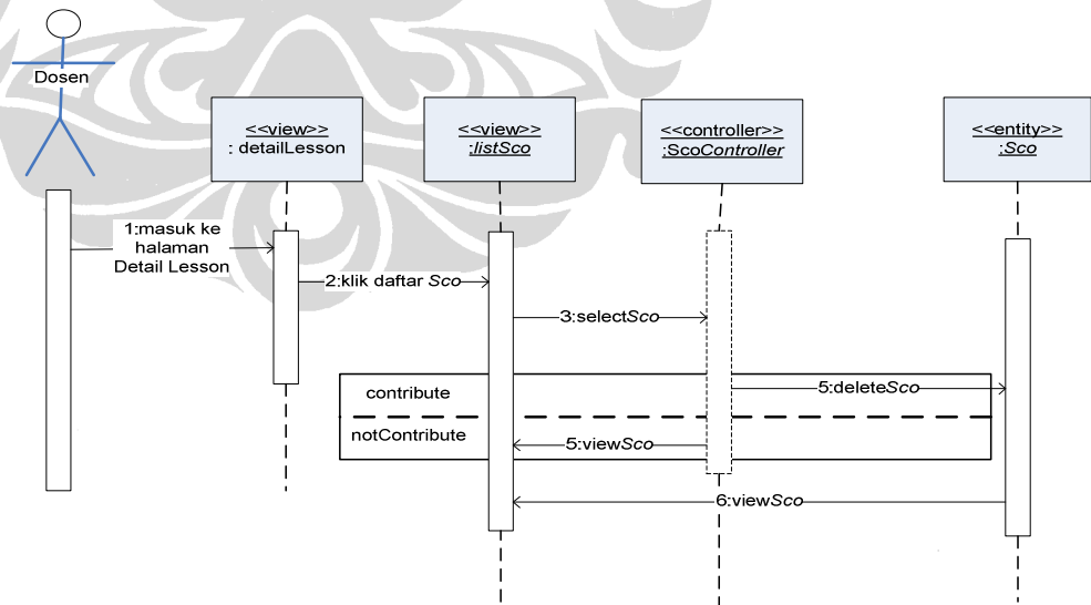
Gambar 63. Sequence diagram untuk use case delete Sco
