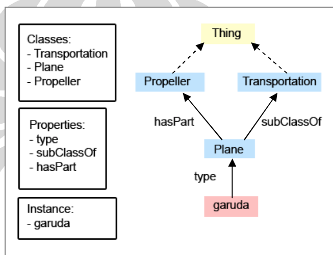
Gambar 3.2 Contoh Ontologi
