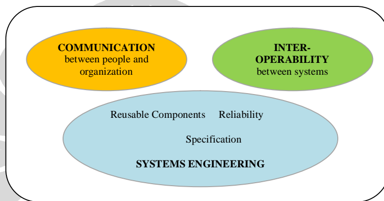
Gambar 3.3 Kegunaan Ontologi
