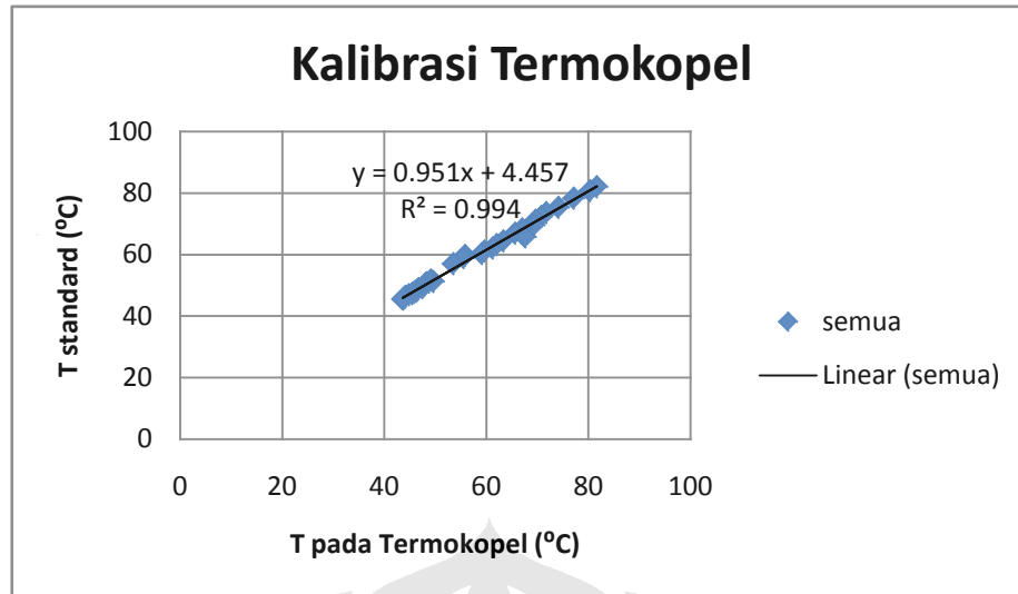
Gambar IV. 11 Hasil kalibrasi termokopel
