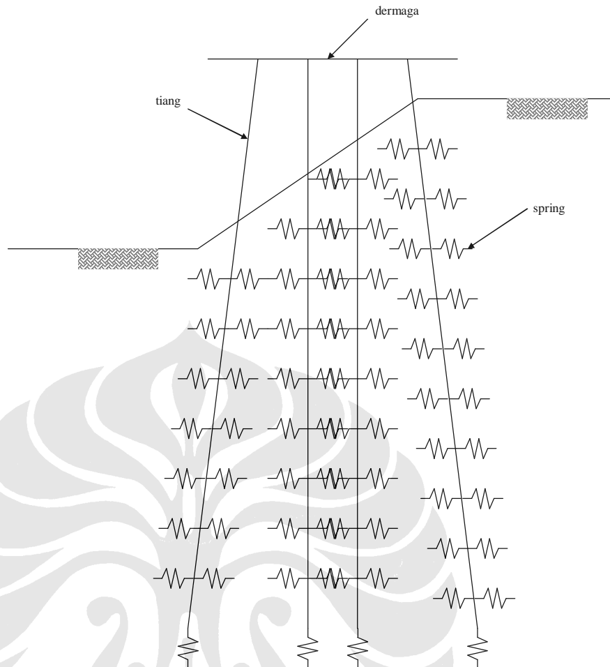
Gambar 2. 18 Modelisasi Struktur dalam Program SAP2000
