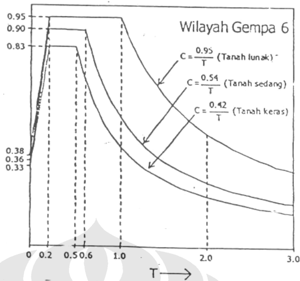
Gambar 2. 7. Spektrum Respons Gempa Rencana (Sumber: SNI 03-1726-2002, Perencanaan Ketahanan Gempa untuk Bangunan Gedung)
