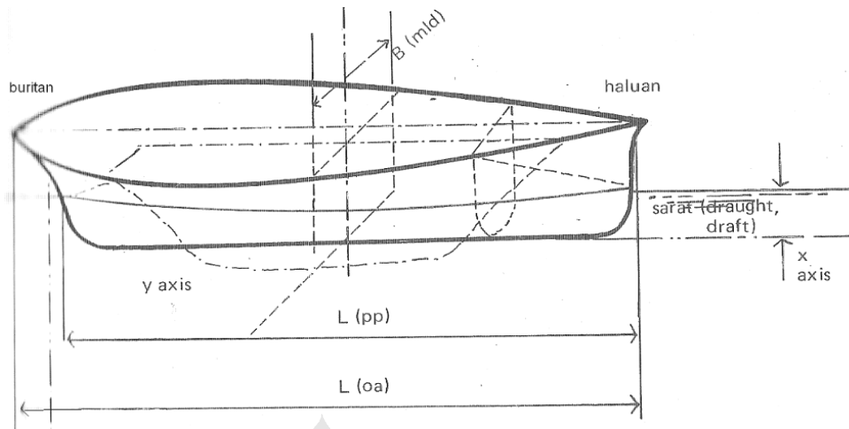
Gambar 2. 2. Dimensi kapal
