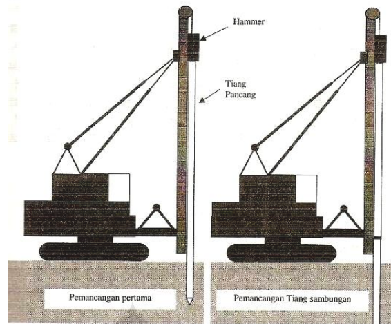
Gambar 2. 19 Proses Pemancangan dan Sambungan
