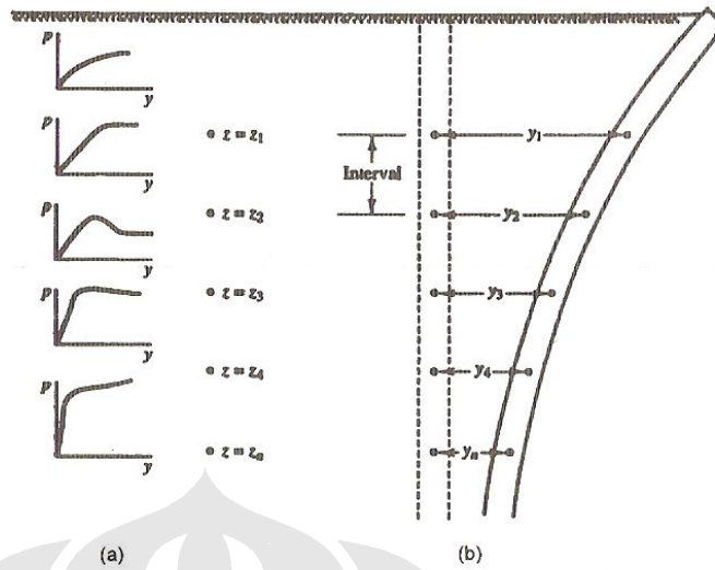
Gambar 2. 11 Konsep Kurva P-y pada Kedalaman Bervariasi
