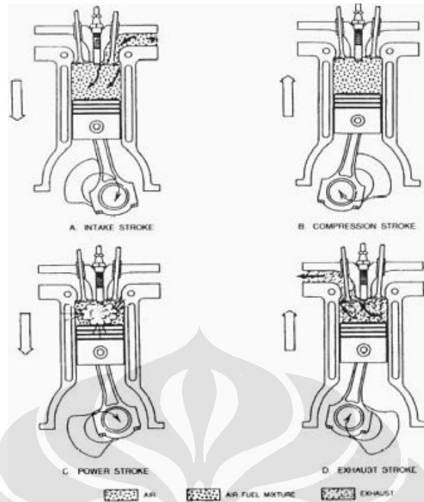
Gambar 2.1. Proses kerja motor Otto empat langkah
