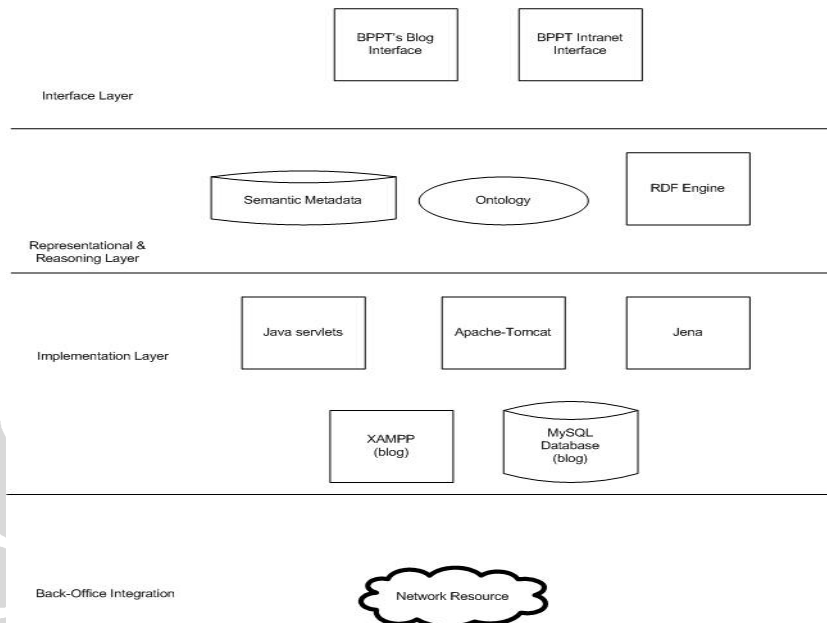
Lampiran A.1 Arsitektur BPPT Intranet
