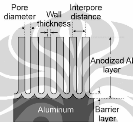
Gambar 2.6. Penampang melintang AAO dengan beberapa parameter untuk karakterisasi [16]
